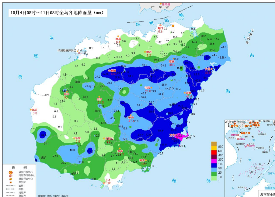
图 1 2024 年 10 月 4 日 08 时~11 日 08 时全岛雨量 (单位:毫米; 图中红色数字为城区测站雨量, 黑色数字为乡镇自动站雨量)
