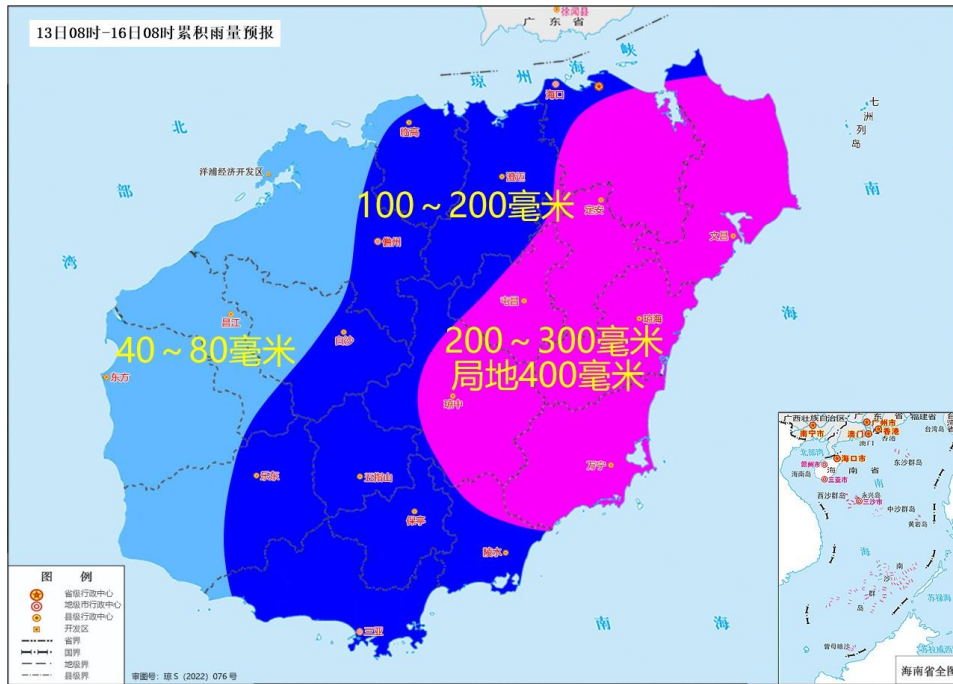
图2 2024年10月13日08时~16日08时雨量预报图(单位:毫米)
