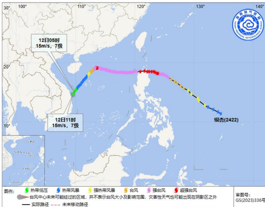
图1 “银杏”11月12日05时预报路径图
