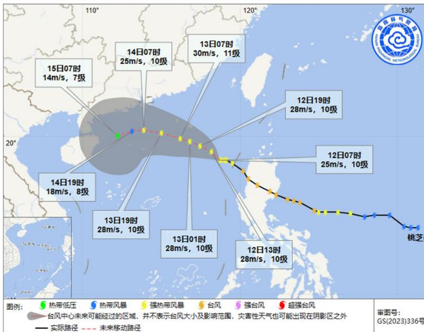
图2 “桃芝”11月12日07时预报路径图
