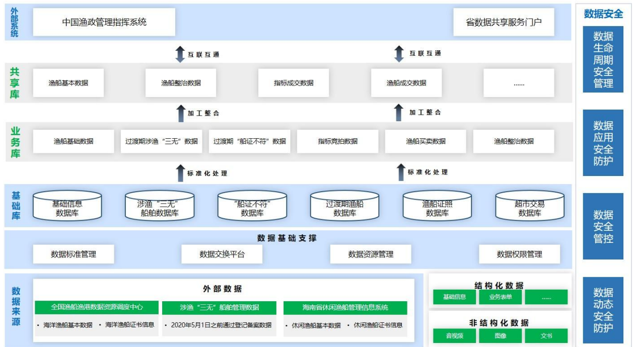
图 数据架构
