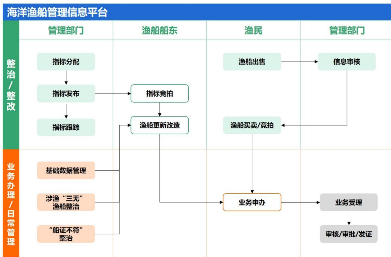
图 业务架构
